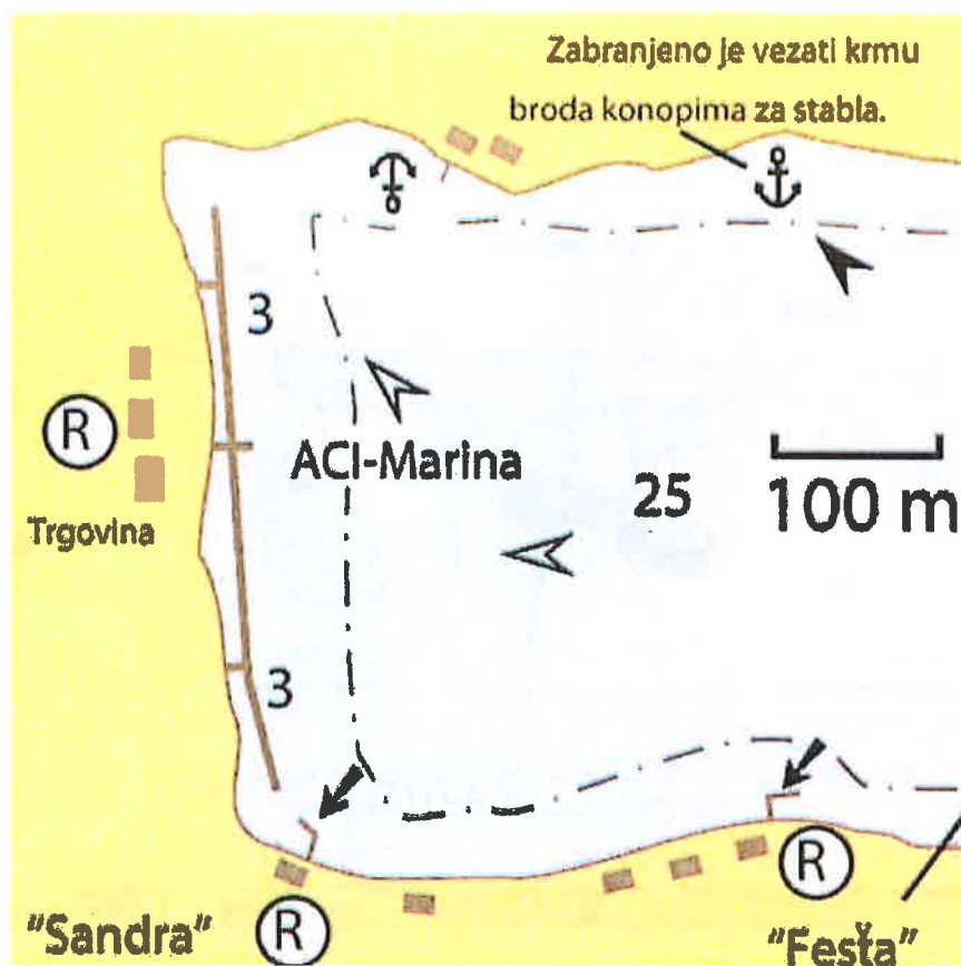
Prilog 1a. Isječak pomorske karte s prilaznim plovnim putem
